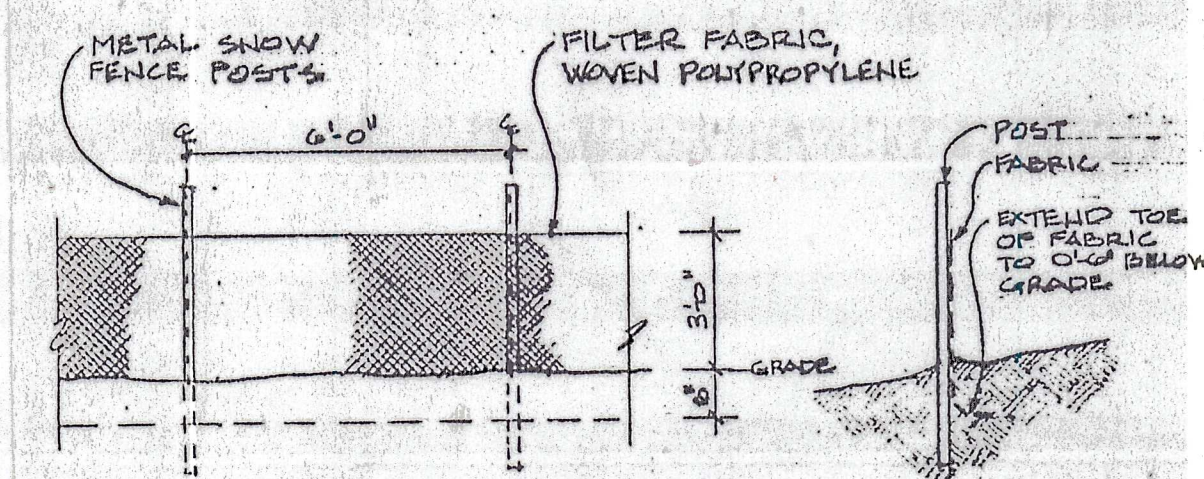
SILTATION FENCE
